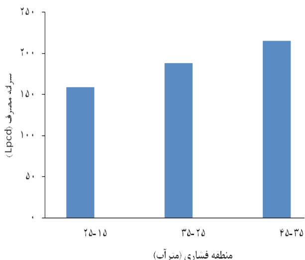
نمودار ۱: سرانه مصرف آب در مناطق فشاری مختلف شهر ازن
