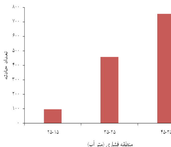
نمودار ۲: اثر میزان فشار بر تعداد حوادث شبکه آب ازنای در سال‌های ۱۳۹۱ تا ۱۳۹۳
