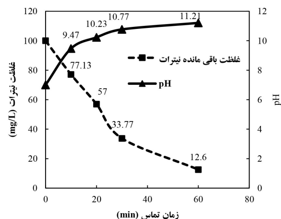
شکل ۲: میزان تغییرات pH و غلظت نیترات در شرایط آزمایش (الف) AC، (ب) DC
