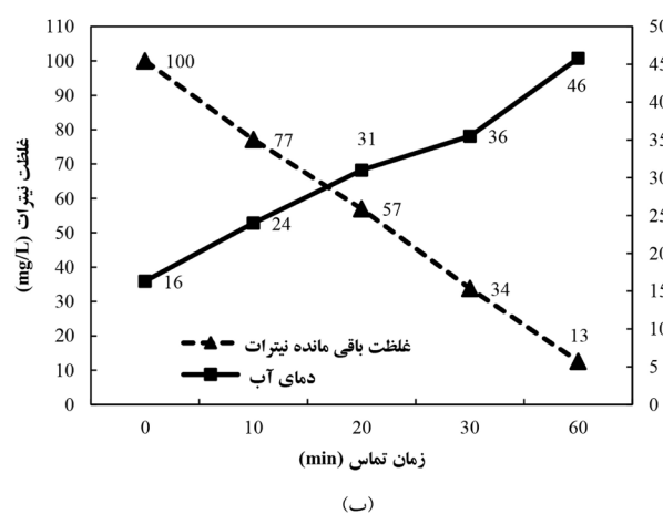
شکل ۴: تغییرات دما و غلظت نیترات در شرایط بهینه الف) AC، ب) DC
