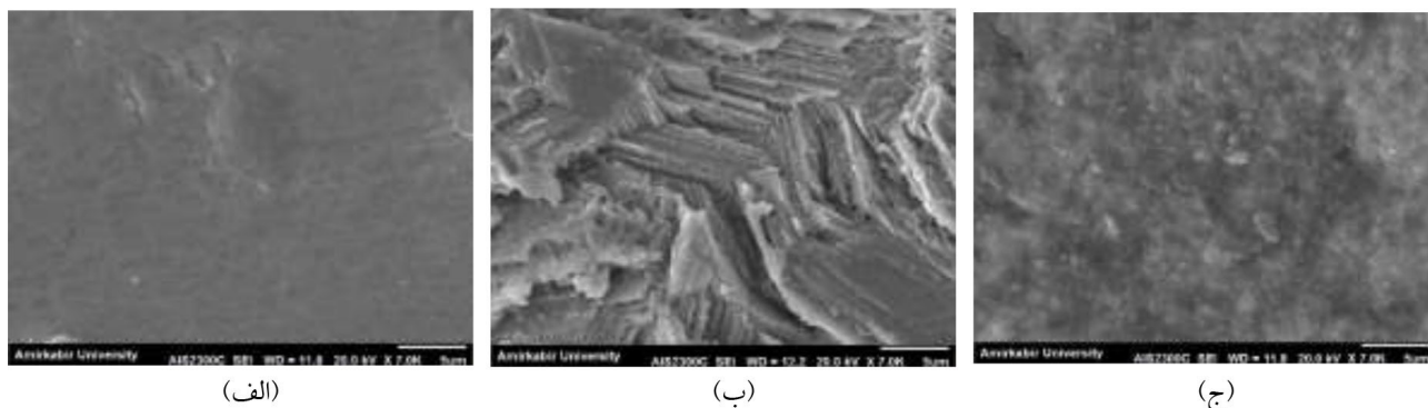
شکل ۶: عکس های SEM الکترود Zn با DC : الف) قبل از استفاده ب) آندی طی فرآیند الکتروشیمیایی ج) کاتدی طی فرآیند الکتروشیمیایی
