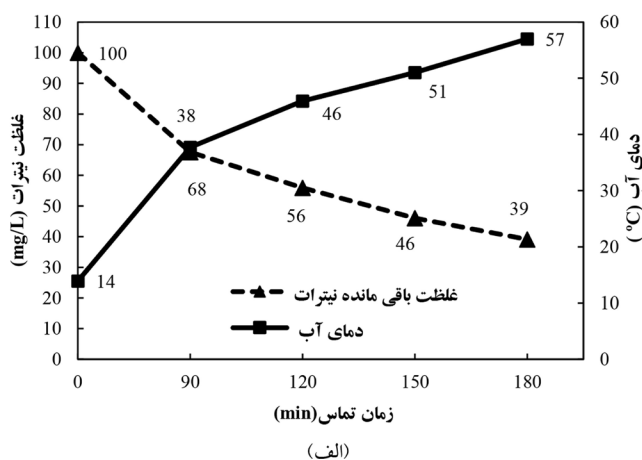
شکل ۴: تغییرات دما و غلظت نیترات در شرایط بهینه الف) AC، ب) DC
