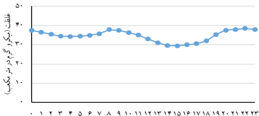
نمودار ۴: تغییرات میانگین ساعتی غلظت ذرات معلق PM_{2.5} میکرون در مشهد در سال ۱۳۹۵
