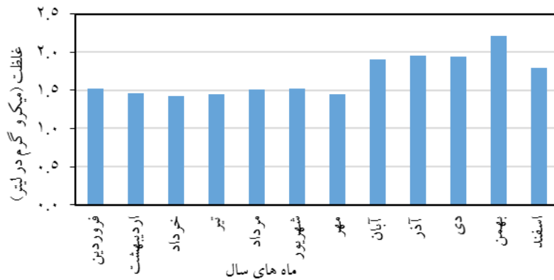
نمودار ۲: تغییرات میانگین ماهانه غلظت منوکسید کربن در مشهد در سال ۱۳۹۵
