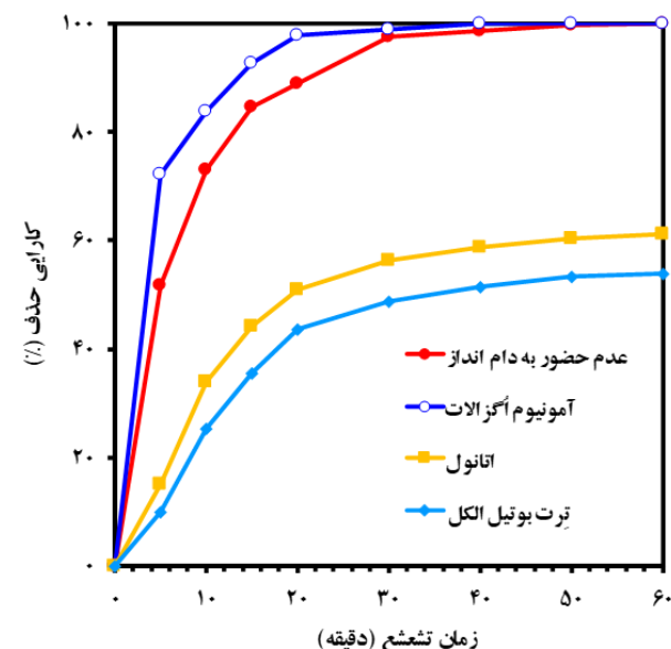
نمودار ۱۱. تاثیر اسکانوجره‌های رادیکالی بر کارایی حذف فتوکاتالیستی رنگ اسید رد ۱۴ (غلظت اولیه رنگ اسید رد ۱۴ برابر با 20 \text{ mg L}^{-1} ، مقدار اولیه نانوکامپوزیت برابر با 0.4 \text{ g L}^{-1} pH اولیه برابر با ۳)
