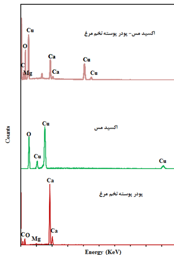
نمودار ۲. تصویر EDX از نمونه‌ها
