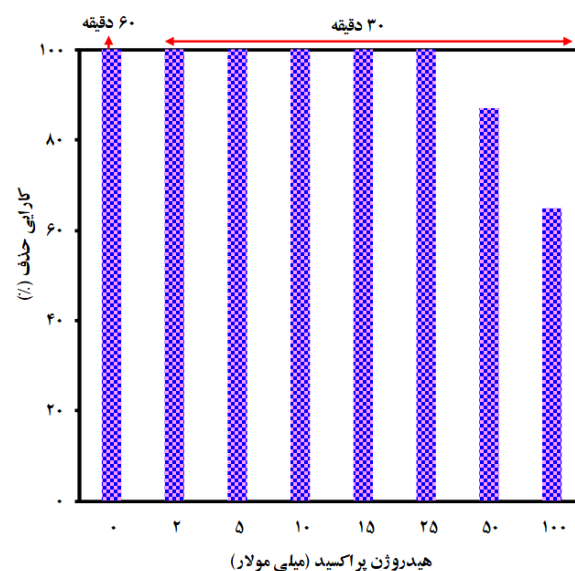
نمودار ۷: تأثیر غلظت اولیه هیدروژن پراکسید بر کارایی حذف فتوکاتالیستی رنگ اسید رد ۱۴ (غلظت اولیه رنگ اسید رد ۱۴ برابر با ۲۰ \text{ mg L}^{-1} ، مقدار اولیه نانوکامپوزیت برابر با ۰/۴ \text{ g L}^{-1} ، \text{pH} اولیه برابر با ۳، زمان تماس برابر با ۳۰ دقیقه).
