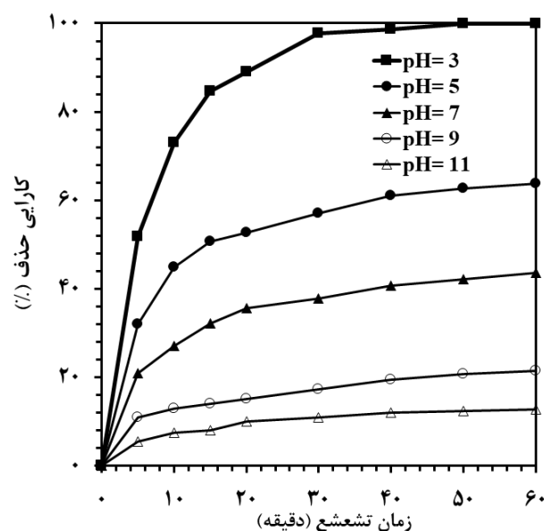
نمودار ۳. تأثیر pH اولیه بر کارایی حذف فتوکاتالیستی اسید رد ۱۴ (غلظت اولیه رنگ اسید رد ۱۴ برابر با 20 \text{ mg L}^{-1} ، مقدار اولیه نانوکامپوزیت برابر با 0.4 \text{ g L}^{-1} )
