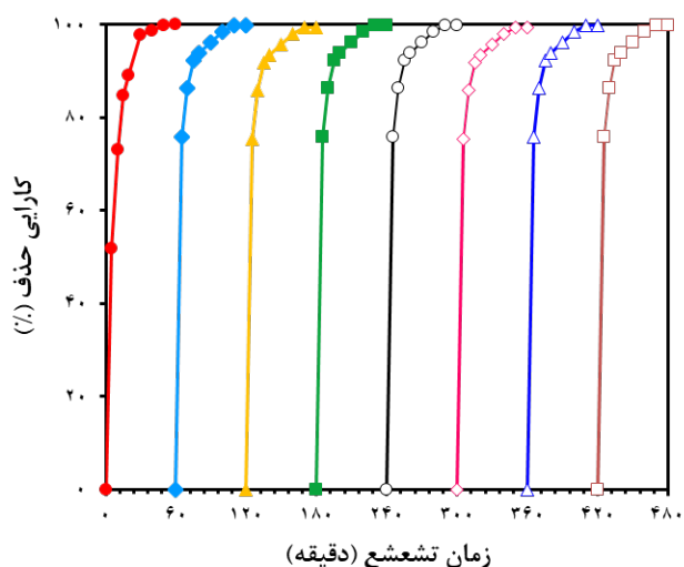
نمودار ۱۲. کارایی نانوکامپوزیت بازیافت شده بر حذف فتوکاتالیستی رنگ اسید رد ۱۴ (غلظت اولیه رنگ اسید رد ۱۴ برابر با 20 \text{ mg L}^{-1} ، مقدار اولیه نانوکامپوزیت برابر با 0.4 \text{ g L}^{-1} pH اولیه برابر با ۳)
