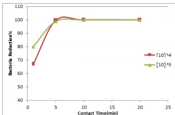
شکل ۳: تأثیر زمان تماس بر راندمان گندزدایی ازن با دوز ۳ میلی گرم در لیتر و تعداد باکتری های ۱۰ ۴ و ۱۰ ۵ CFU/ml
