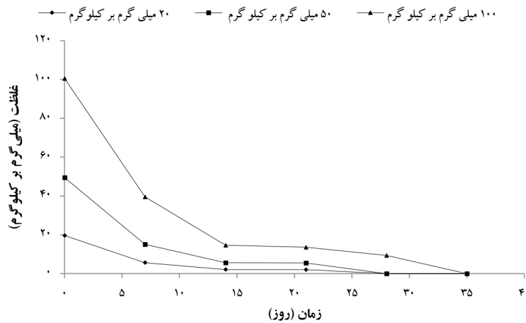
نمودار ۳: تغییرات غلظت C/N در طول فرایند کمپوست‌سازی
