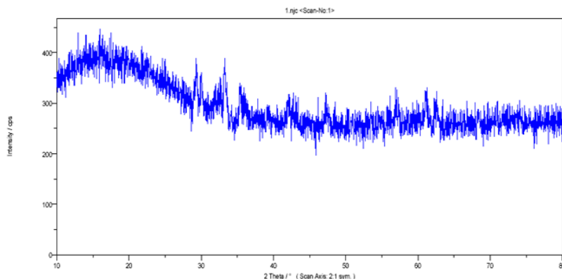
شکل ۱: پراش اشعه ایکس (XRD) سرباره اصلاح‌شده فولاد
