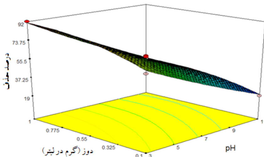
شکل ۲: پاسخ سطحی بازده حذف TCE در برابر دوز nZVI و pH (زمان واکنش = ۷۰ دقیقه و غلظت TCE = ۵۵ میلی گرم در لیتر)
